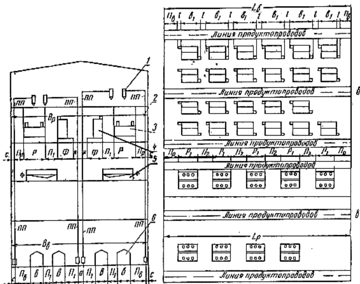
Рис.14 Расположение оборудования в размольном отделении (первый вариант): а - поперечный разрез; б - план вальцового этажа; в - план рассеивного этажа; 1 - циклон-разгрузитель; 2 - продуктопровод; 3 - рассев; 4 - фильтр; 5 - ситовая машина; 6 - вальцовый станок.
