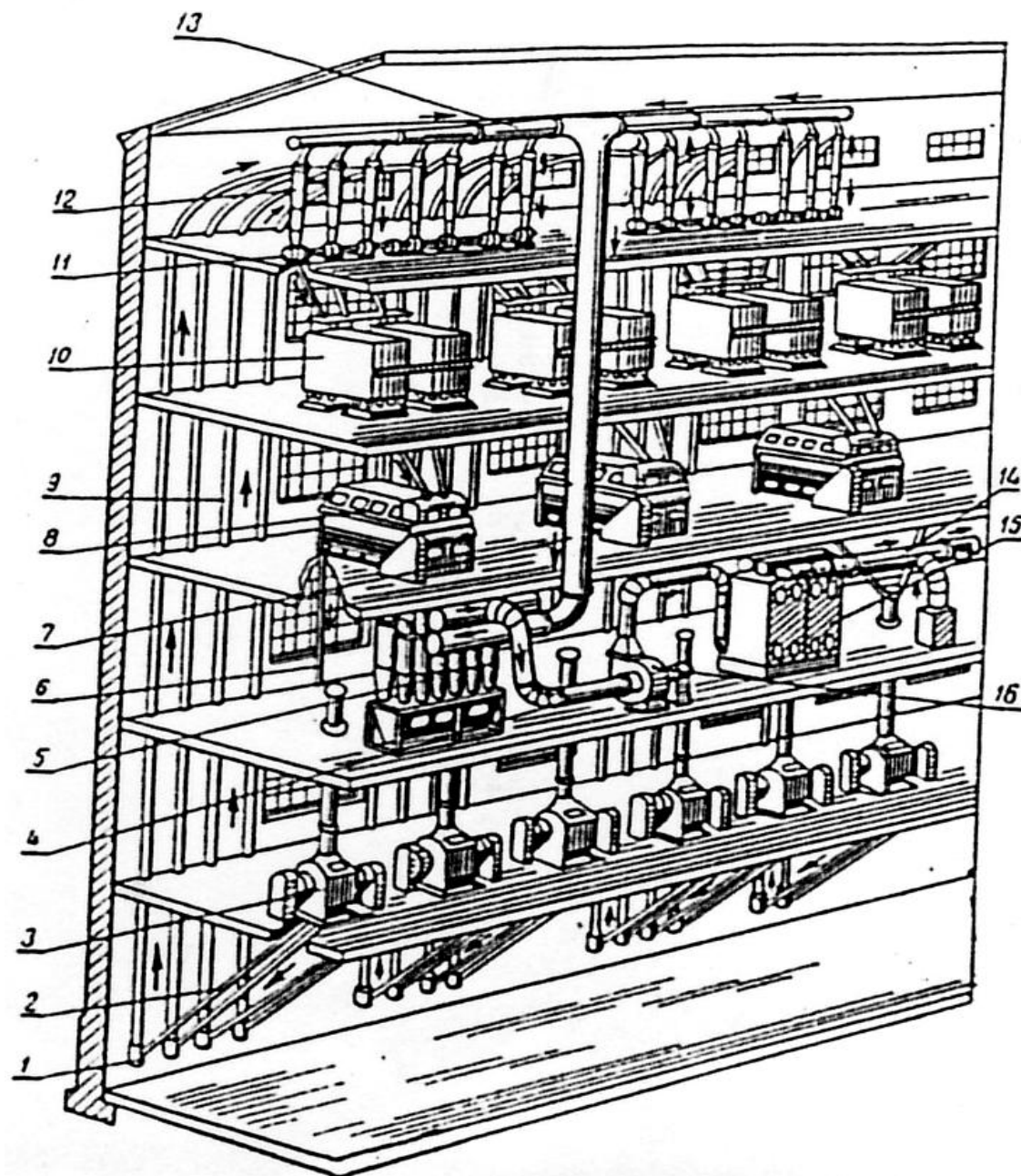
Рис. 13 Размольное отделение мукомольного завода с внутрицеховым пневматическим транспортом продуктов: 1-пневмоприемник; 2,6-самотечные трубы; 3-вальцовый станок; 4,7,13,14-воздухопроводы; 5-циклон; 8-ситовеечная машина; 9-материалопровод; 10-рассев; 11-шлюзовой затвор; 12-разгрузитель; 15-матерчатый фильтр; 16-вентилятор
