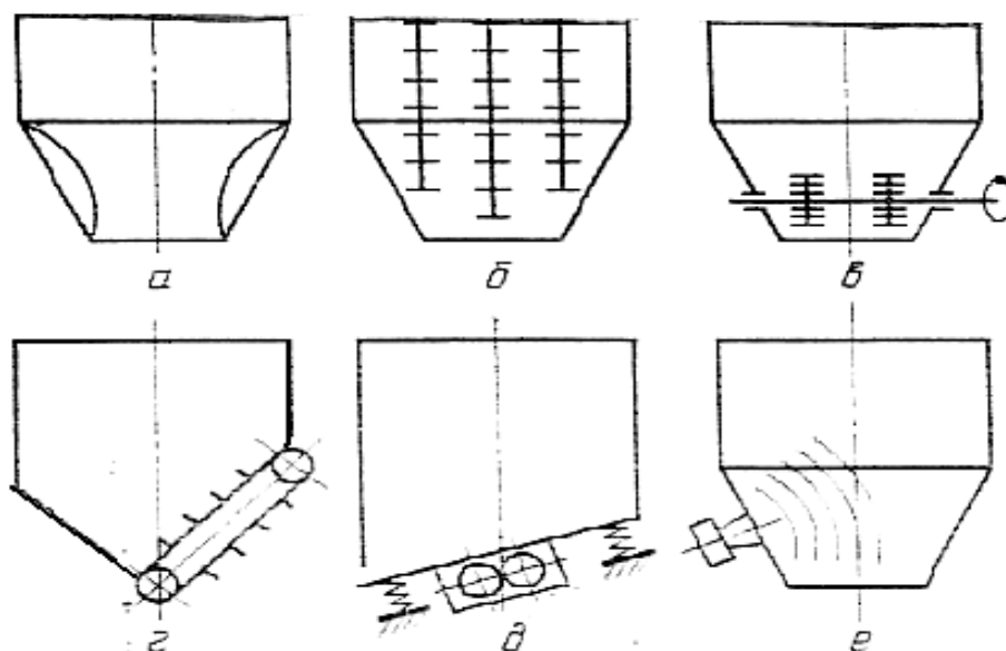
Рис.9 Побудители истечения: а – параболоидальной формы; б – механический штанговый; в – механический ротационный; г – скребковый питатель; д – вибрационный; е – пневматический (азрирование).
